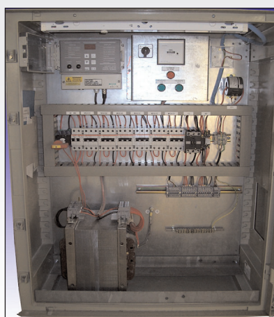
Типовая панель управления
