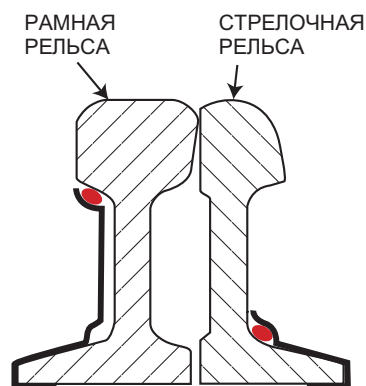
Типовое размещение нагревательных кабелей на рельсах
